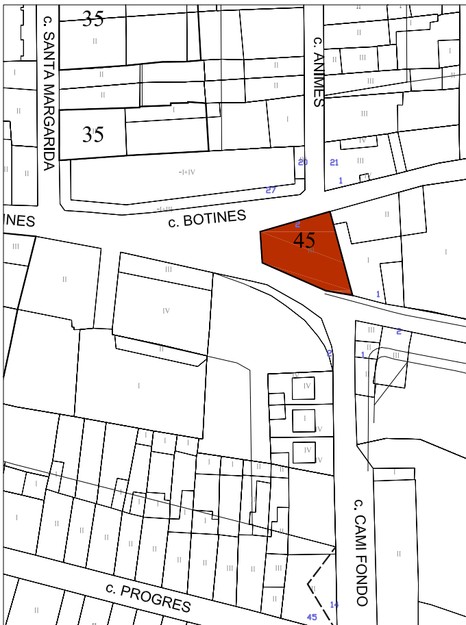
EMPLAÇAMENT E: 1/1000
