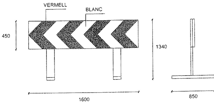
DETALL TANCA DIRECCIONAL ESTRETA
