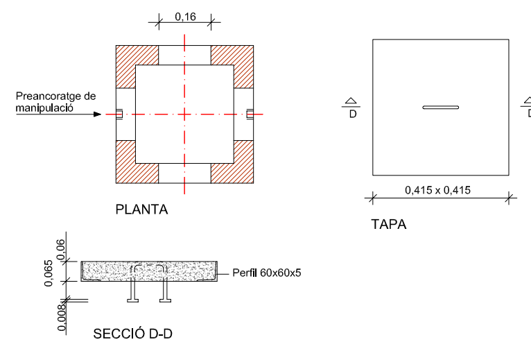
ARQUETA PREFABRICADA DE TELÈFONS TIPUS "HF"
