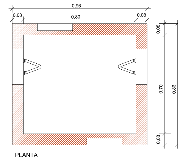
ARQUETA PREFABRICADA DE TELÈFONS TIPUS "HF"
