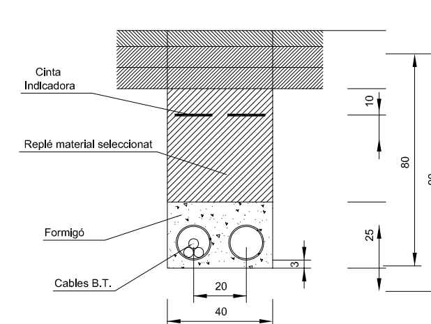
Rasa tipus d'1 circuït sota vial amb tub formigonat
