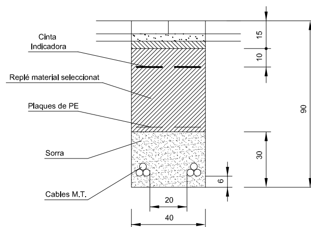
Rasa tipus de 2 circuïts sota vorera protecció amb sorra
