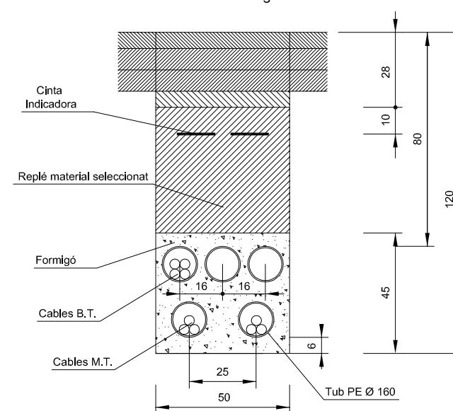
Rasa tipus de 1 o 2 circuïts de MT i fins 3 de BT sota vial amb tub formigonat
