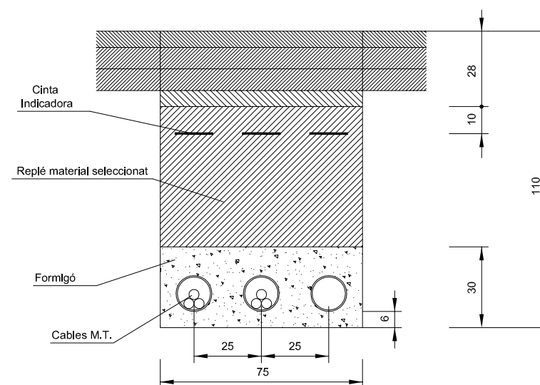
Rasa tipus de 2 circuïts sota vial amb tub formigonat
