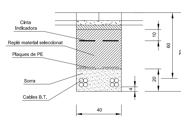
Rasa tipus de 2 circuïts sota vorera protecció amb sorra
