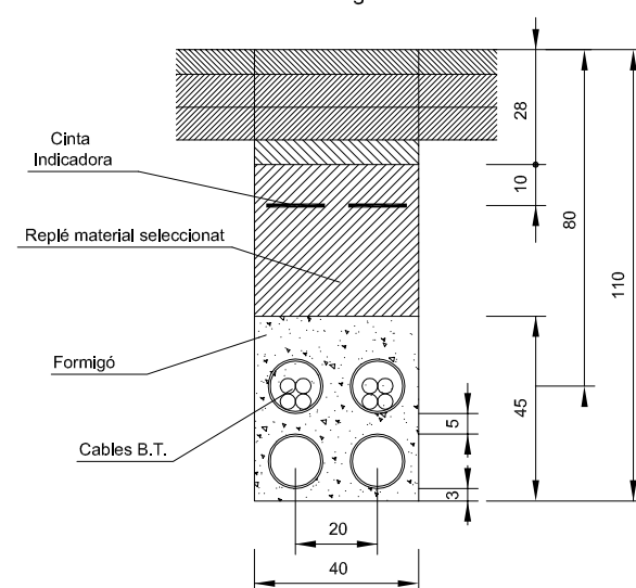
Rasa tipus de 2 circuïts sota vial amb tub formigonat
