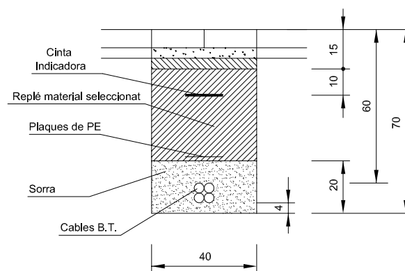
Rasa tipus d'1 circuït sota vorera protecció amb sorra
