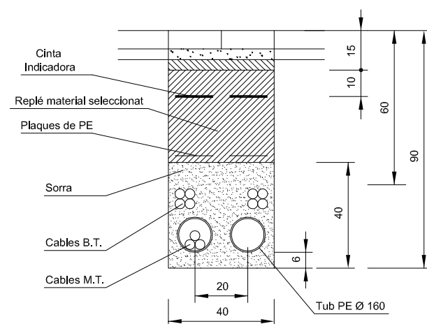
Rasa tipus de 1 o 2 circuïts sota vorera protecció amb sorra
