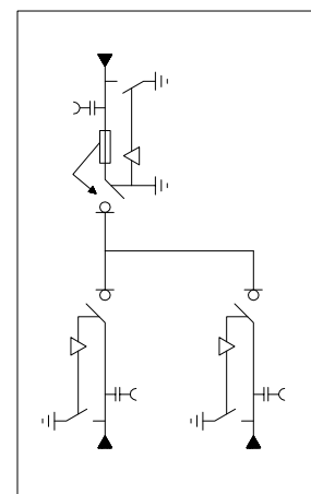
ESQUEMA UNIFILAR
