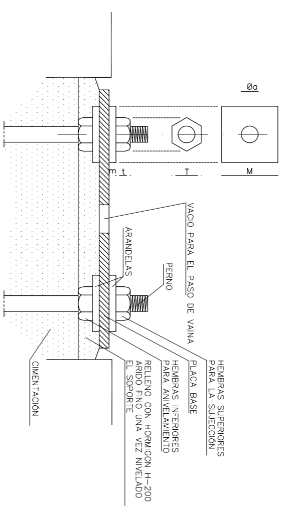
BASE TIPO
